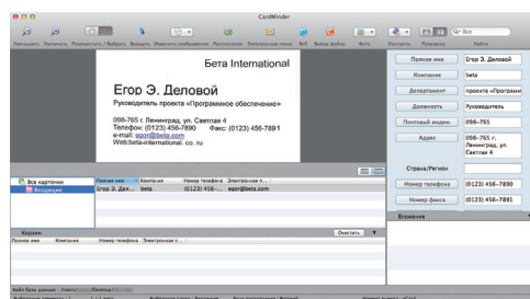
Окно CardMinder
